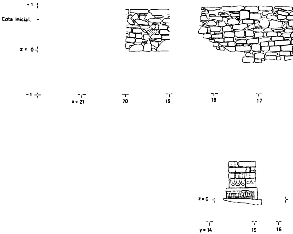
6. Plano VI: Alzado de la cimentación del muro norte: VI-1. Pared norte. VI-2. Contrafuerte postizo, alzado este. VI-3. Contrafuerte este, alzado este. VI-4. Contrafuerte central, alzado este. VI-5. Contrafuerte central, alzado oeste. VI-6. Contrafuerte oeste, alzado oeste.
